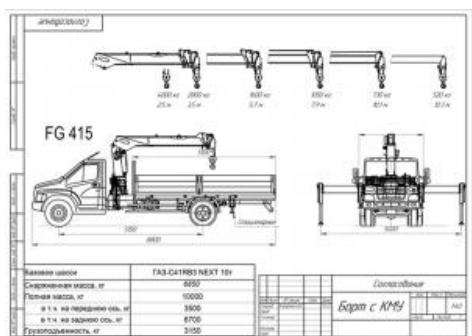
Манипулятор ГАЗон NEXT с КМУ FG 415
